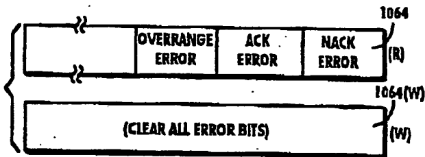
Fig. 37G ERROR REGISTER
